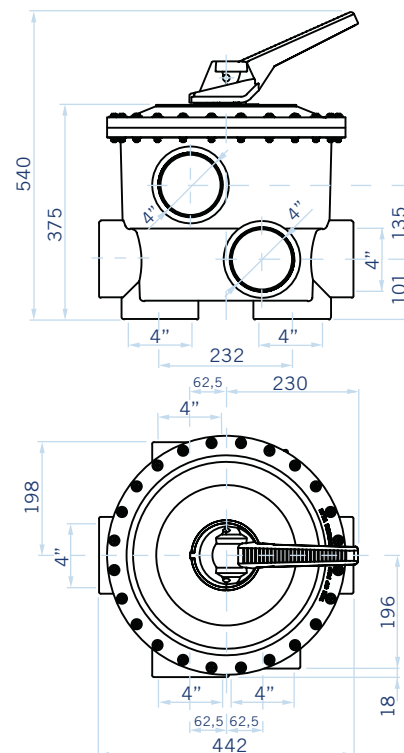
Modelo 4". Código 33933 Model 4". Code 33933
