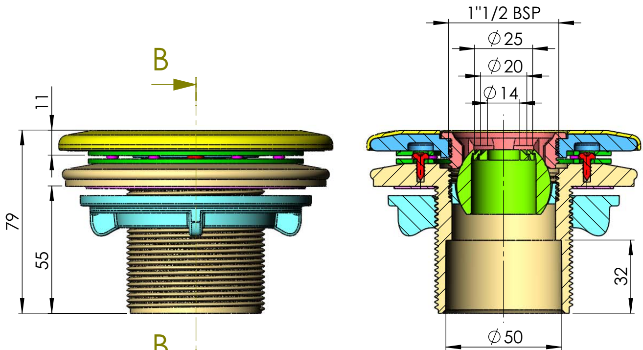
SECCIÓN B-B
